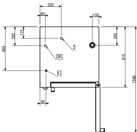
Felülnézet
